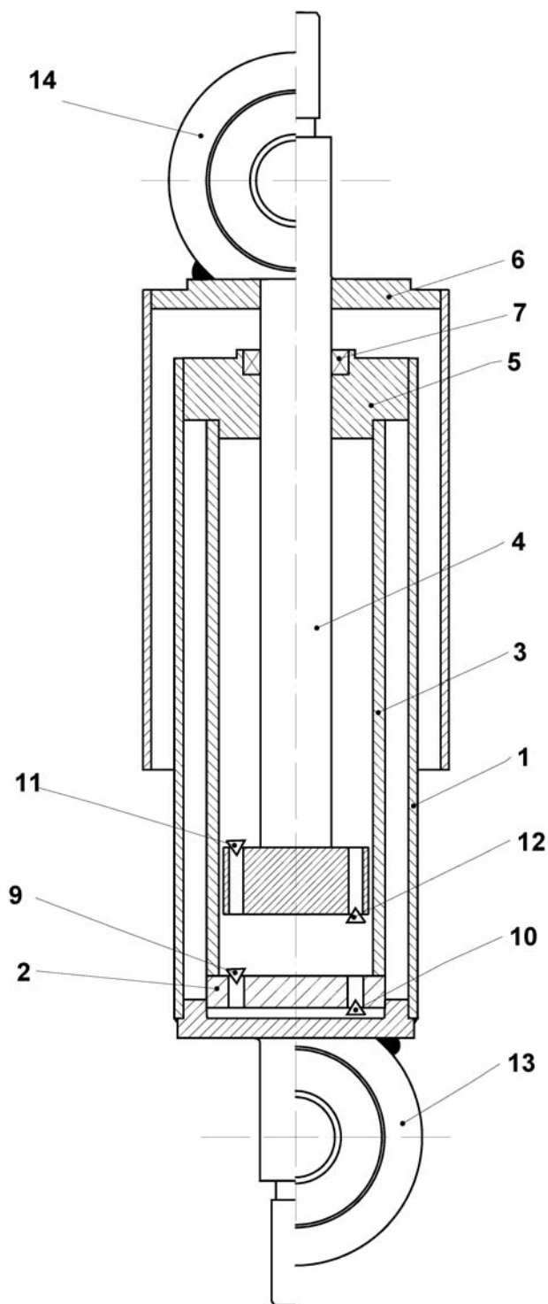
Figura 1*) — Schema de principiu a unui amortizor hidraulic
