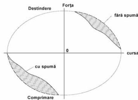
Figura 4*) — Influența formării spumei asupra diagramei de reglaj
