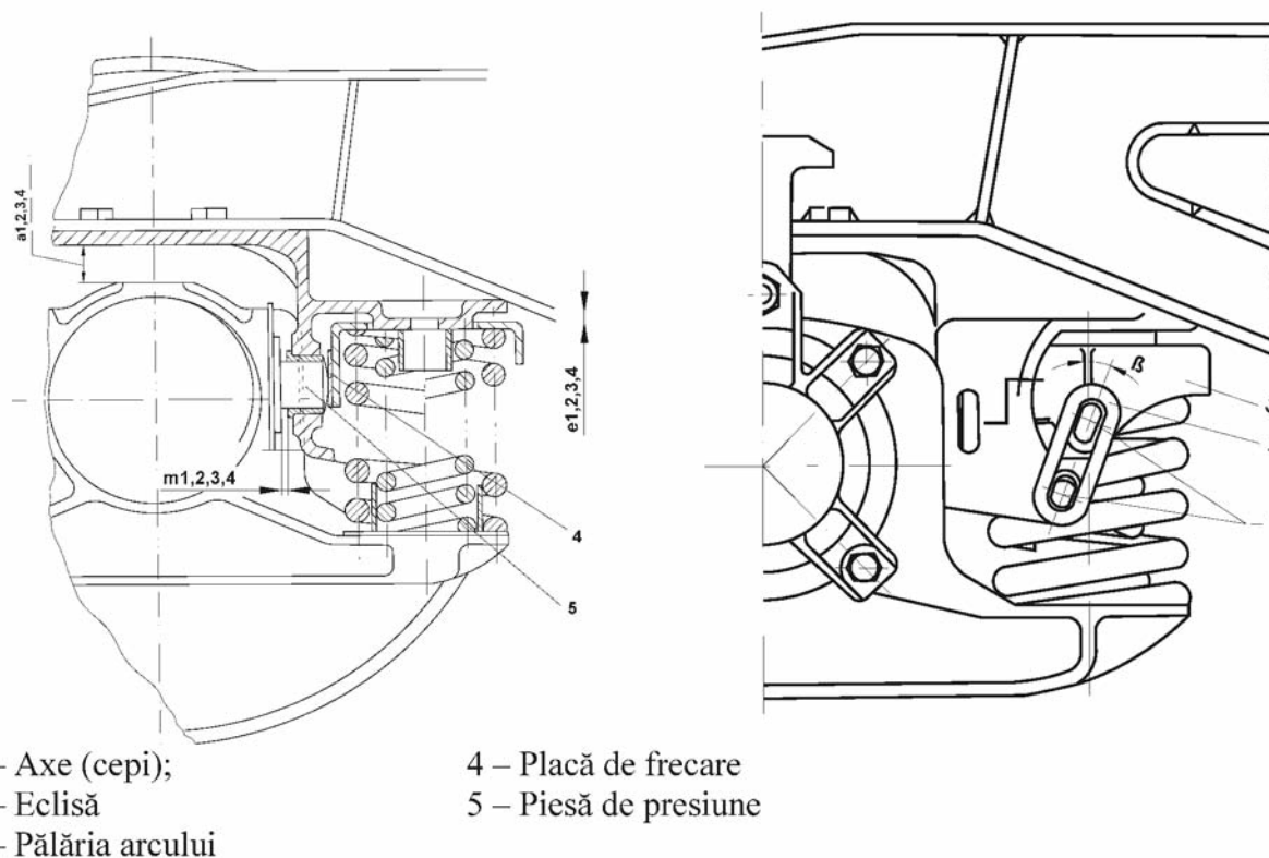
Figura 13*) — Amortizor cu fricțiune pentru vagoanele de marfă echipate cu boghiu Y25. Schemă de principiu
