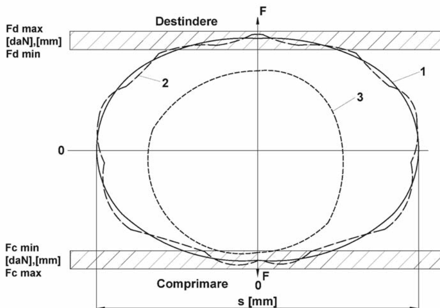
Figura 2*) — Diagramă de reglaj (model)
