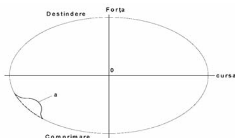
Figura 7*) — Influența arcului supapei de admisie asupra diagramei de reglaj
