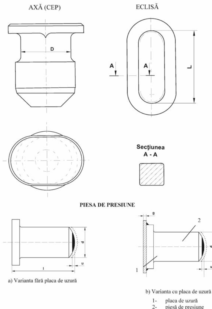
Figura 15*) — Cotele care indică zonele cu uzuri ale axelor (cepilor), eclisei și piesei de presiune
