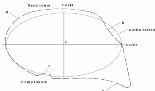
Figura 6*) — Influența reglării supapelor de admisie și comunicare și a cantității de ulei asupra diagramei de reglaj
