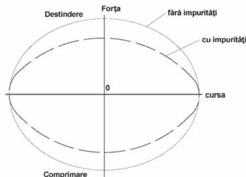
Figura 5*) — Influența prezenței impurităților din ulei asupra diagramei de reglaj
