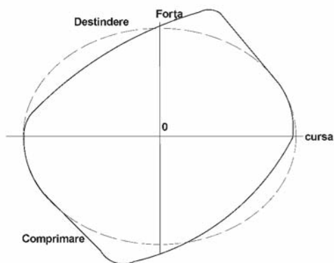
Figura 9*) — Influența uzurii și a elasticității elementelor de cauciuc ale prinderilor asupra diagramei de reglaj
